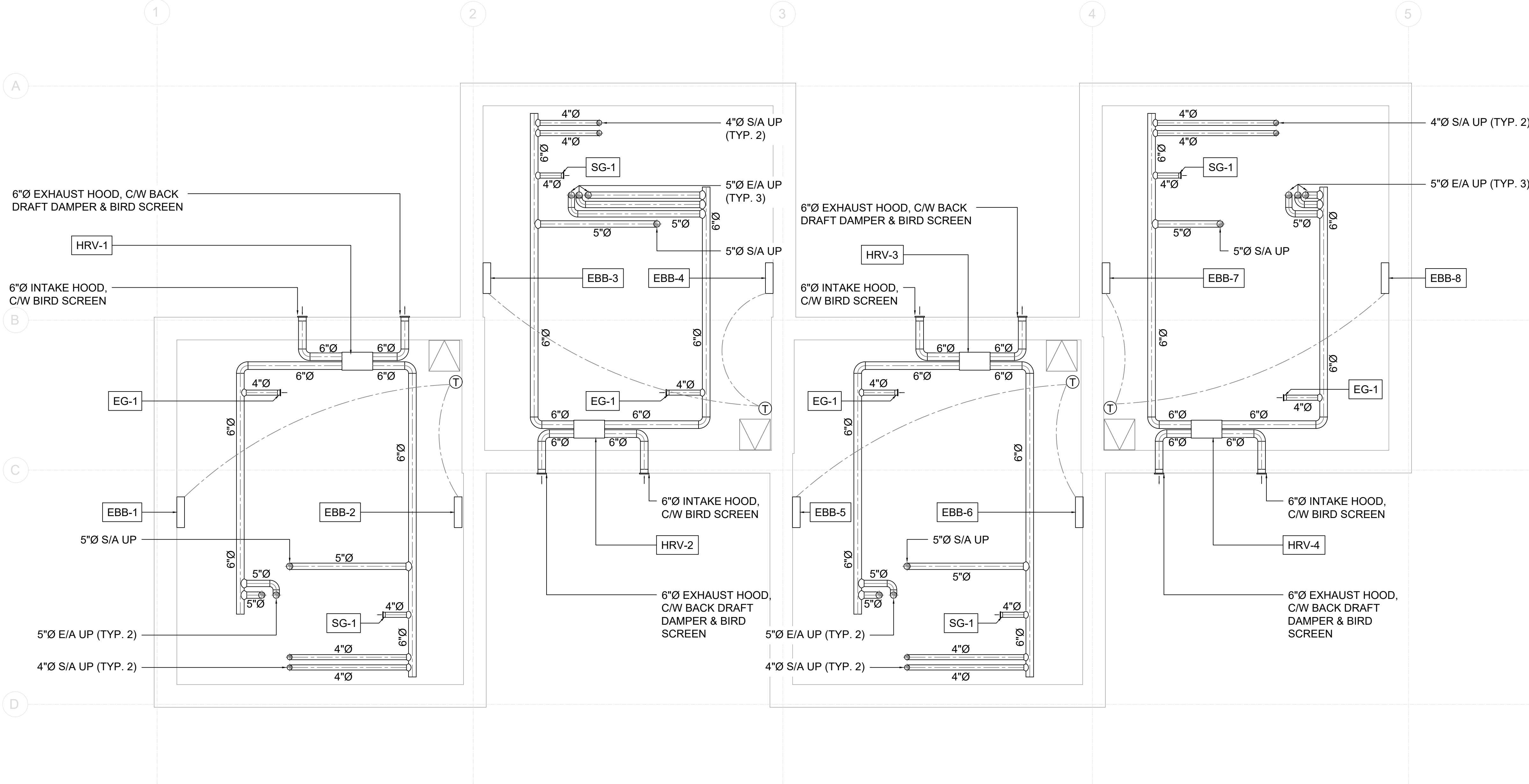
M0 1 CRAWL SPACE PLAN 1/4" : 1'
